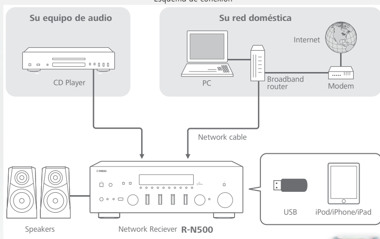
Esquema de conexión
